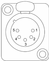
XLR 5FEM
